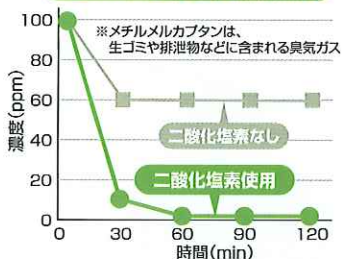
メチルメルカプタンの消臭試験
