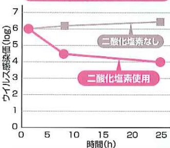
ウイルスIの除去試験
